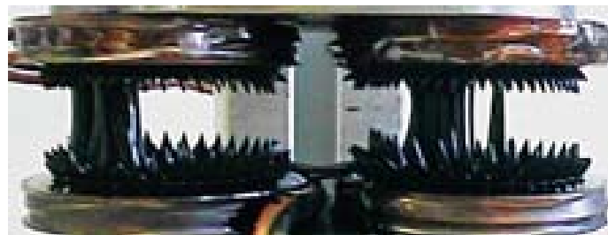
80 mT_Magnetfluid – Säulenbildung und „Spikes“ im Magnetfeld zwischen Elektromagneten
